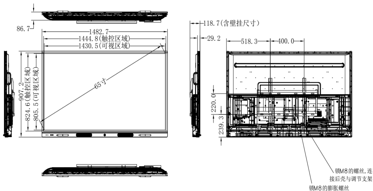
六视图
