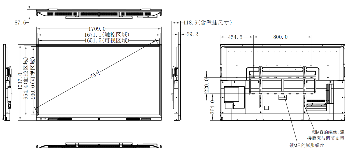
六视图
